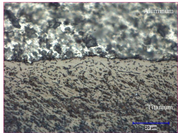
Figure 2. Aluminum-titanium diffusion couples
